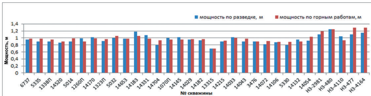
Рис. 4. Несоответствие мощностей по данным разведки и горных работ. Шахта “Юбилейная”
